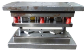
Press Tools
